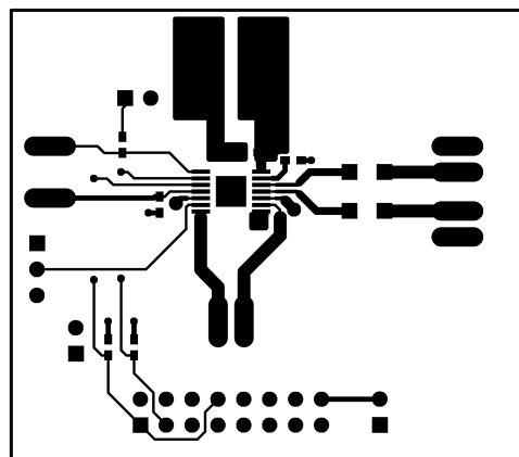
Figure 19. Top Layer
