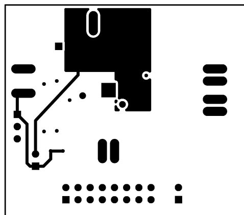
Figure 21. Layer 3
