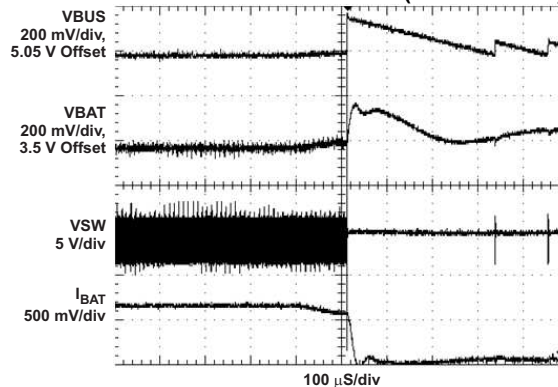
Figure 16. V_{BUS} = 5.05 , V_{BAT} = 3.5\text{ V} , I_{BUS} = 360\text{--}0\text{ mA}
