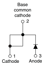
VS-60EPU02PbF
