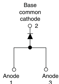
VS-60APU02PbF
